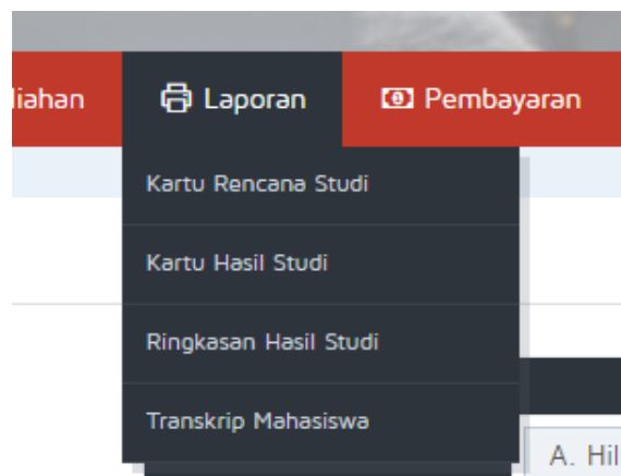
Gambar 4.1 Cetak Laporan
